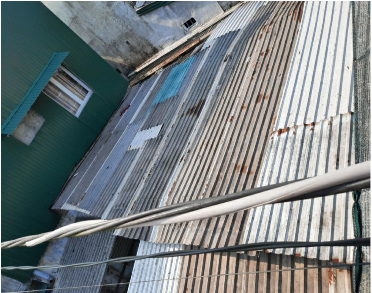
Hình ảnh : Tại vị trí đường dây sau khi đã được xử lý bằng ống bọc cách điện polyme.
